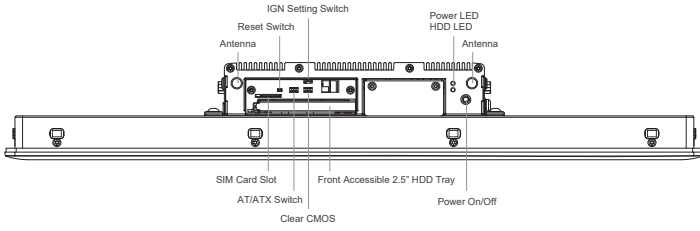
Left I/O
