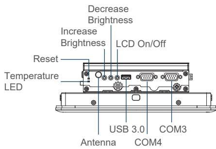
Left I/O
