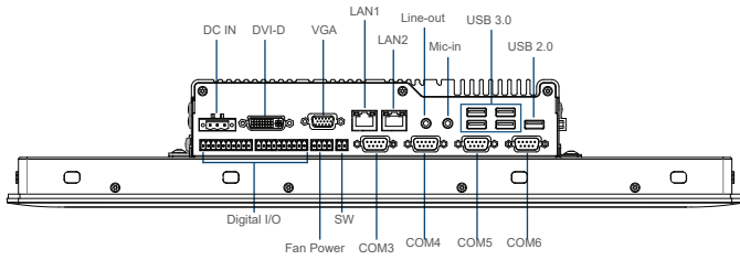
Left I/O
