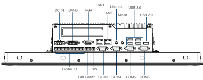
Left I/O
